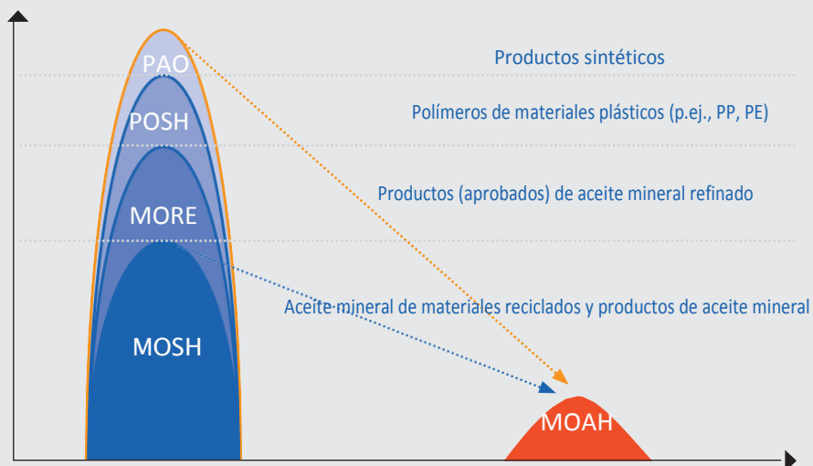
Figura 2: Cambio de la relación MOSH: MOAH comúnmente encontrada en el aceite mineral por MORE, POSH y PAO como análogos de MOSH [de acuerdo con 14 y 15] (para las abreviaturas, ver definiciones y texto)
